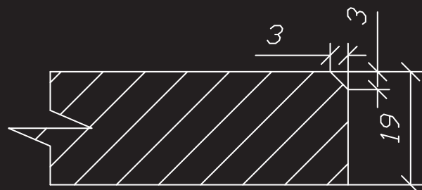
Варіант фрезерування торців №15
