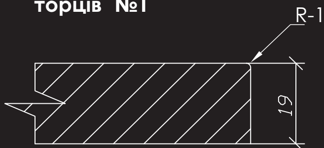
Варіант фрезерування торців №1
