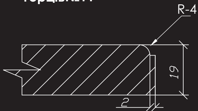
Варіант фрезерування торців №12
